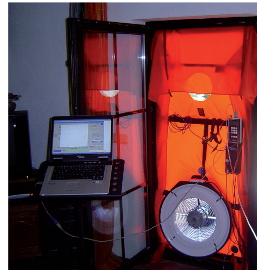
Realización del test de Blower Door [VAND arquitectura]
